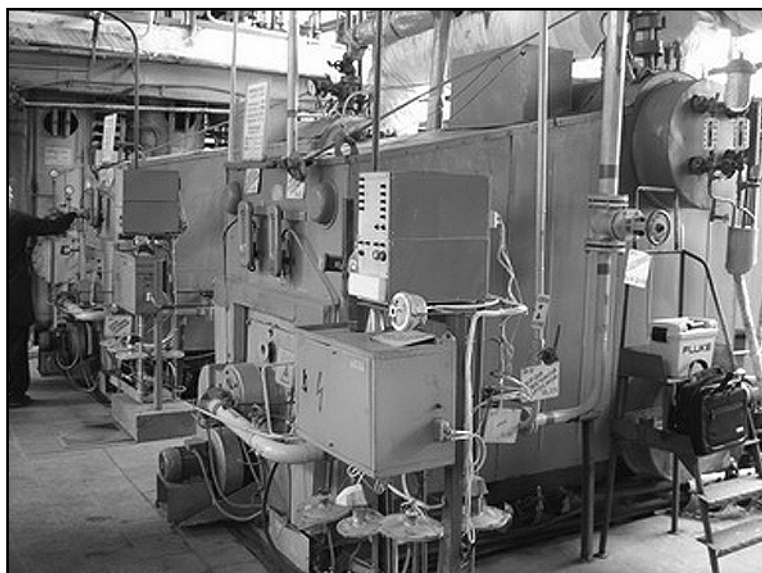
Un alt proiect MoSEFF constă în înlocuirea unui cazan de abur de tip vechi cu unul de abur moderne.
