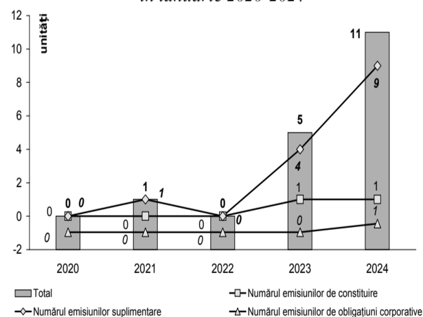
Diagrama nr. 2 Numărul emisiunilor de valori mobiliare în ianuarie 2020-2024
