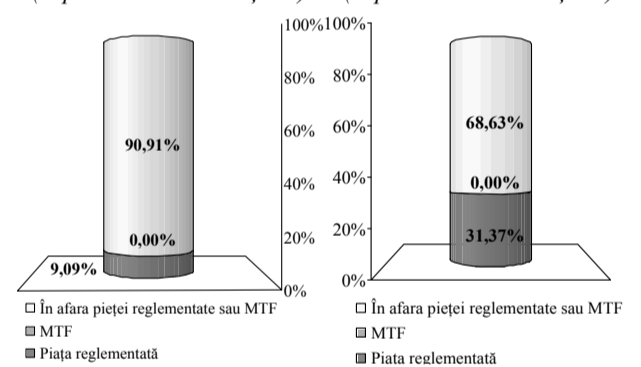
Diagrama nr. 5 Structura tranzacțiilor efectuate în afara pieței reglementate sau MTF în luna ianuarie 2024
