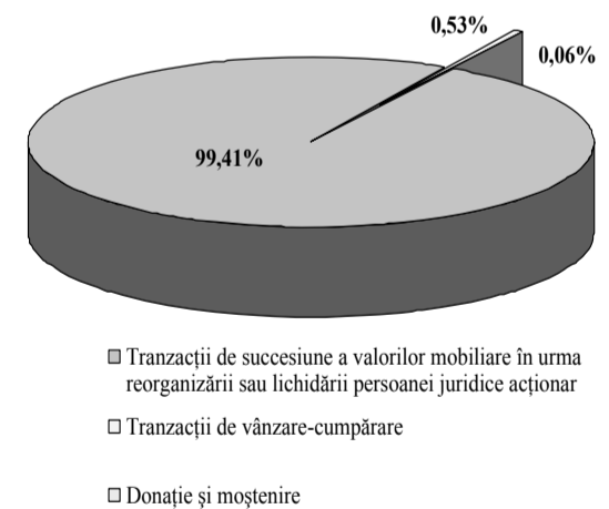
Diagrama nr. 5 Structura tranzacțiilor efectuate în afara pieței reglementate sau MTF în luna ianuarie 2024
