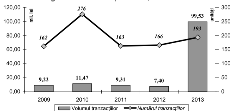
Diagrama nr. 6 Tranzacții extrabursiere, mai 2009-2013
